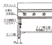
■NEW/パワークック ガステーブル(立消え安全装置搭載タイプ)[新ユニバーサルバーナー搭載]仕様表(RGT-S)
