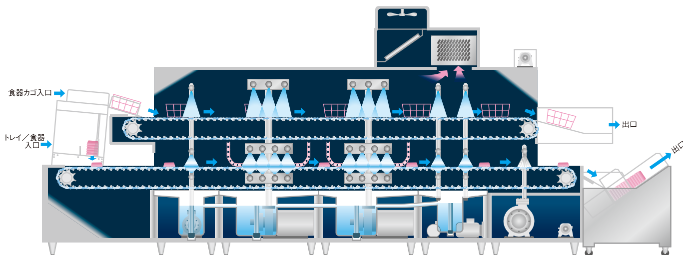
洗浄レーン入口(左)と出口(右)
