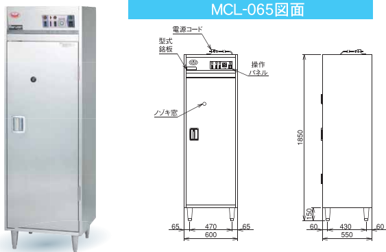
MCL-065図面
