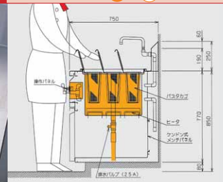
配置 D-D
