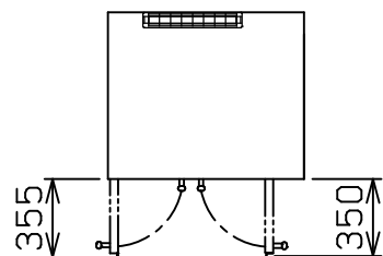
オ - ブン扉開時寸法
